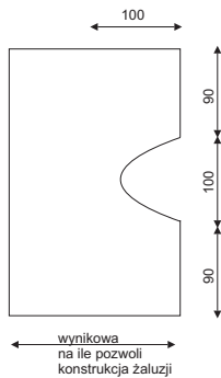
Szkic wyglądu przegród o grubości 8 mm
